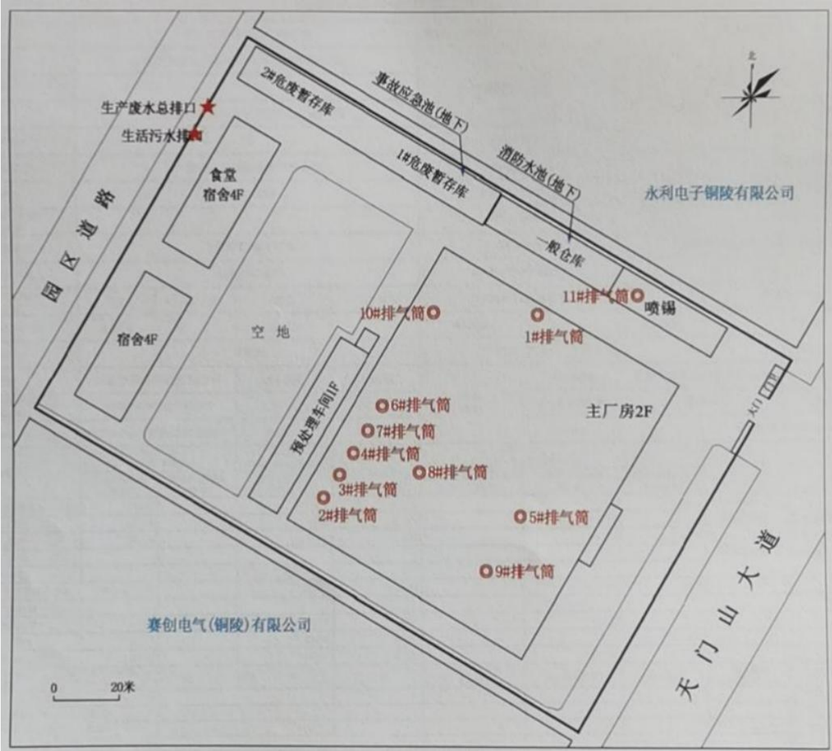
图4.2-1厂区平面布置图
