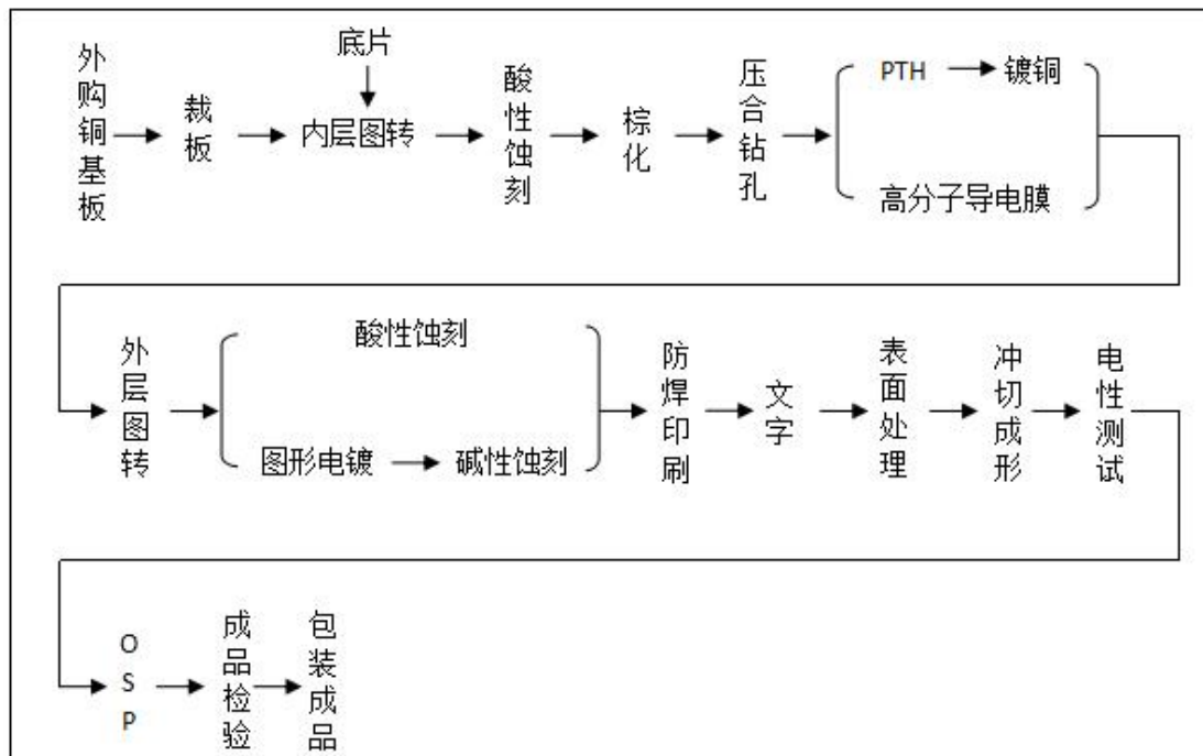
图4.1-1 厂区现有项目总体生产工艺流程图
